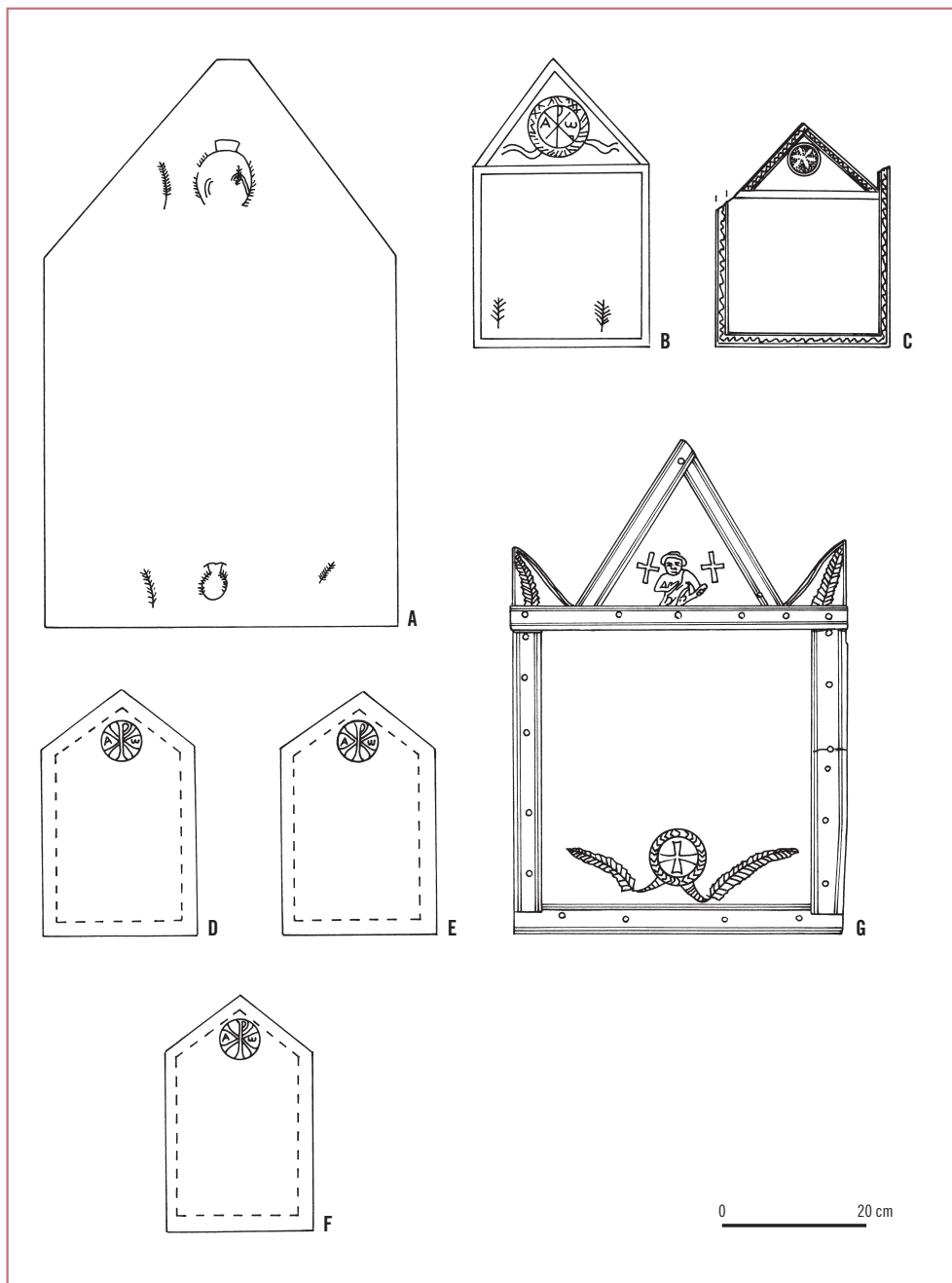
fig. 1. Dibujo de los soportes de las tábulas de patronato con texto de carácter honorífico: A. Tábula de Italica (CIL XII 1856). B. Tábula de Thamugadi (AE 1913, 25). C. Tábula de Sasamón (CIL II 5812). D. Tábula de la ciuitas Senonum (CIL XIII 921a). E. Tábula de la ciuitas Autessiodurensium (CIL XIII 921b). F. Tábula de la ciuitas Aurelianorum (CIL XIII 921c). G. Tábula de Minturnae (AE 1954, 27).
